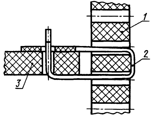
1 — гибкая матрица; 2 — хомут; 3 — ячейка
