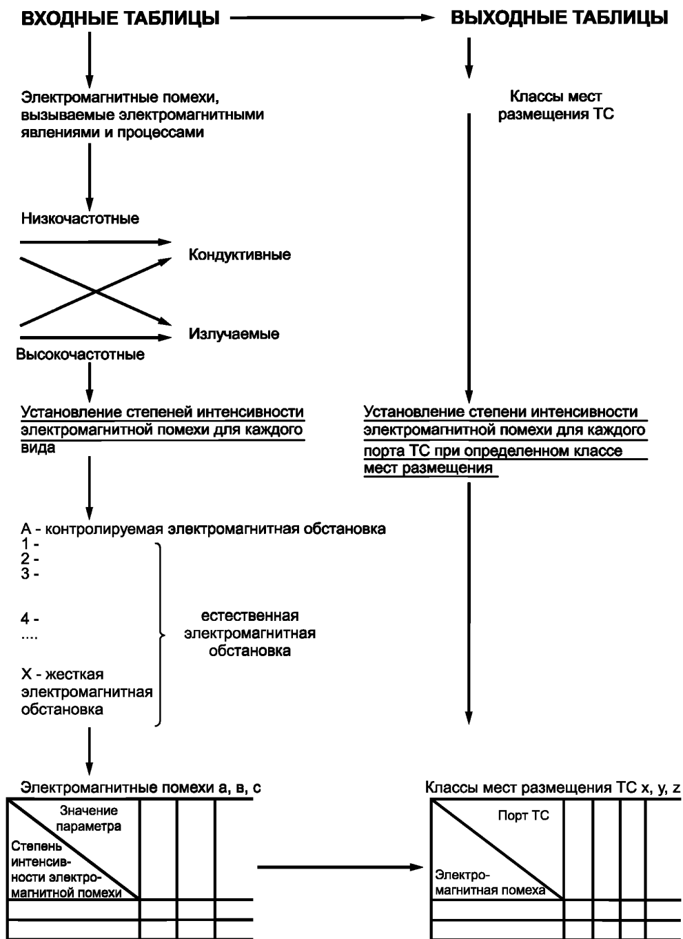
Рисунок 1 — Принципы классификации электромагнитной обстановки
