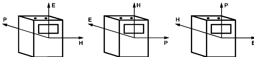
Е — вектор электрического поля; H — вектор магнитного поля; P — направление распространения электромагнитного поля
