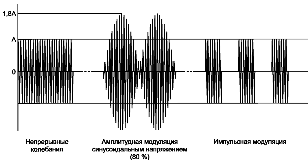
Рисунок 3 — Виды модуляции
