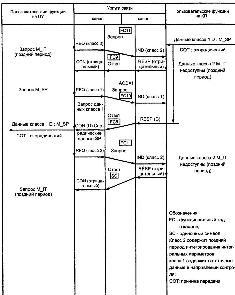
Рисунок 29 — Последовательная процедура, взаимодействие процедур опроса и спорадической передачи однопозиционной информации
