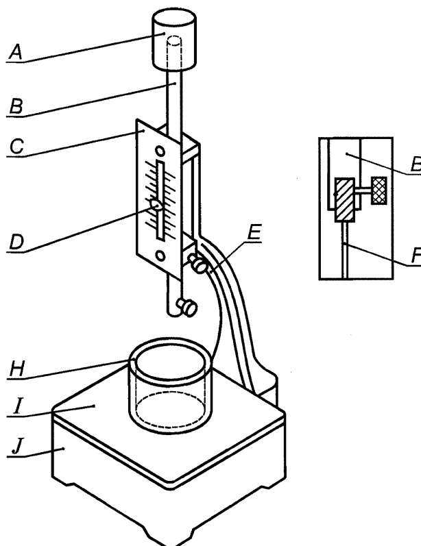
Рисунок 1 — Схема прибора Вика
