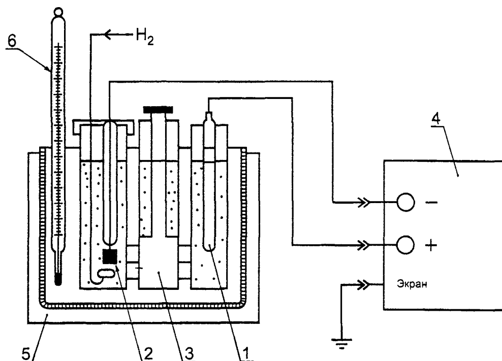
1 — эталонный электрод сравнения; 2 — водородный электрод; 3 — электролитический ключ; 4 — милливольтметр; 5 — термостат; 6 — термометр
