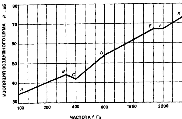
Рис. 2. Расчетная частотная характеристика
