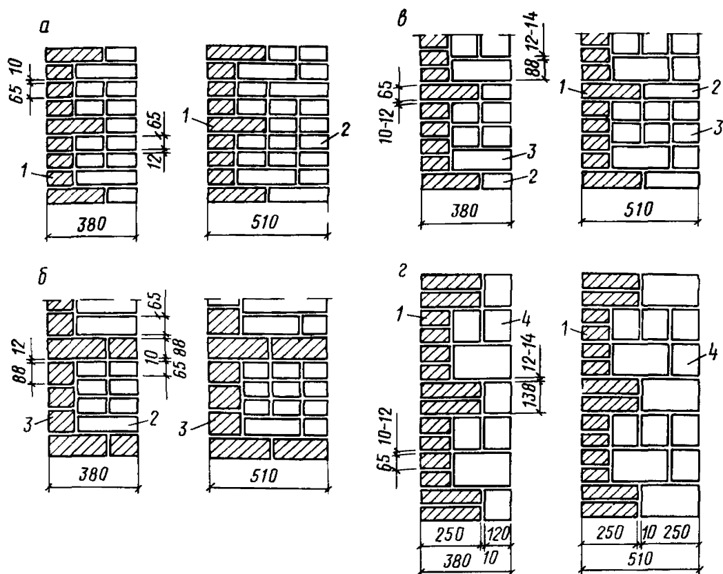
Рис. 1. Облицовка лицевым кирпичом стен
