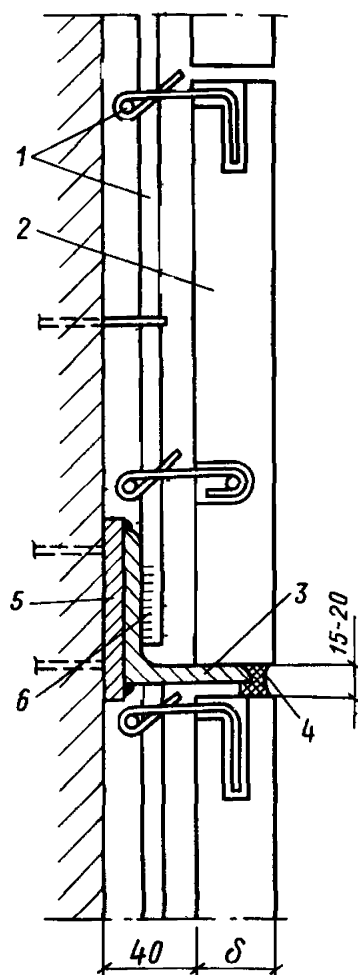
Рис. 6. Вариант устройства компенсационного шва 1 — рабочая арматура; 2 — опорный ряд облицовочных плит; 3 — опорный уголок; 4 — компенсационный шов, 5 — закладная деталь; 6 — рабочая арматура приваривается к уголку
