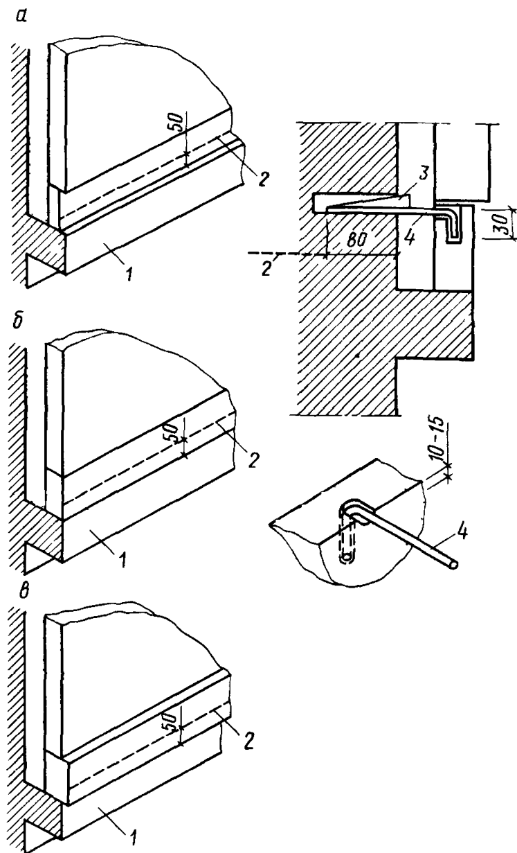
Рис. 7. Облицовка цоколя здания плитами а — западающими за плоскость стены; б — расположенными в плоскости стены; в — выступающими за плоскость стены; 1 — опора; 2 — уровень отмостки; 3 — стальной клин; 4 — крюк
