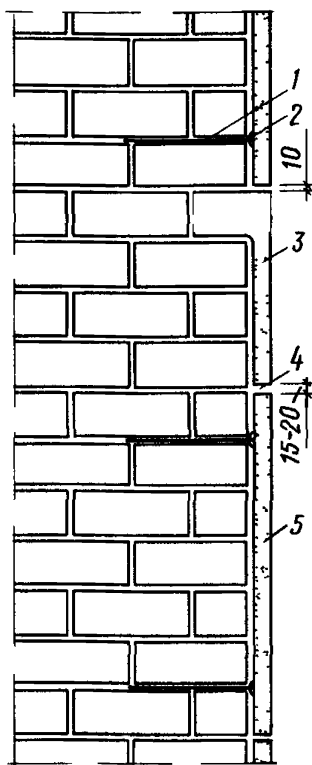
Рис. 12. Кладка из кирпича или камней с облицовкой фасадными бетонными плитами 1 — анкер \phi 4–5 мм; 2 — петля \phi 4 мм; 3 — Г-образная плита; 4 — компенсационный шов; 5 — фасадная плита
