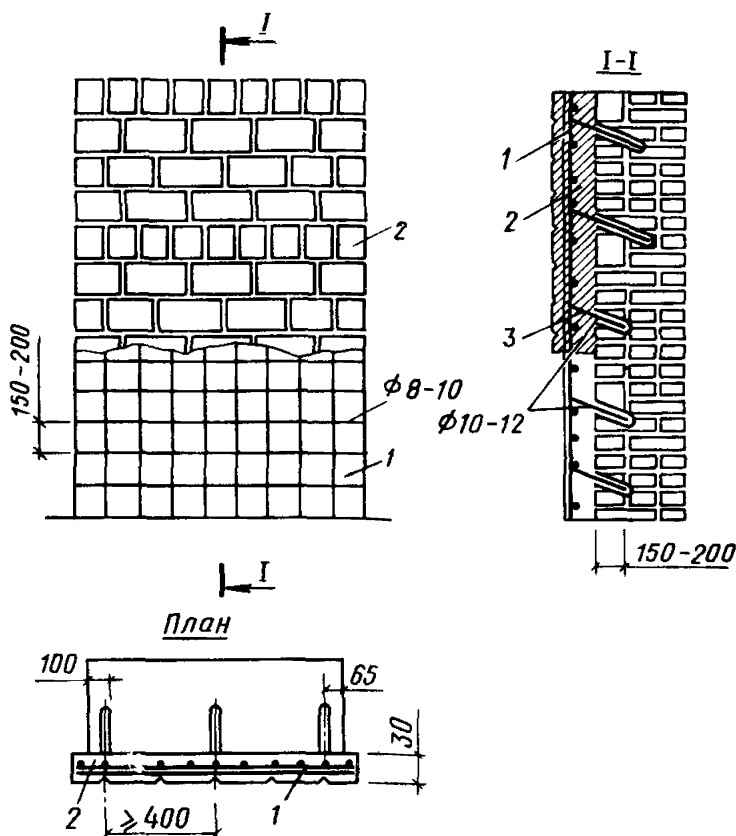
Рис. 17. Пример усиления простенка путем замены разрушенной облицовки железобетонной стенкой 1 — арматурная сетка; 2 — бетон марки 100; 3 — стержни для закрепления сетки к стене
