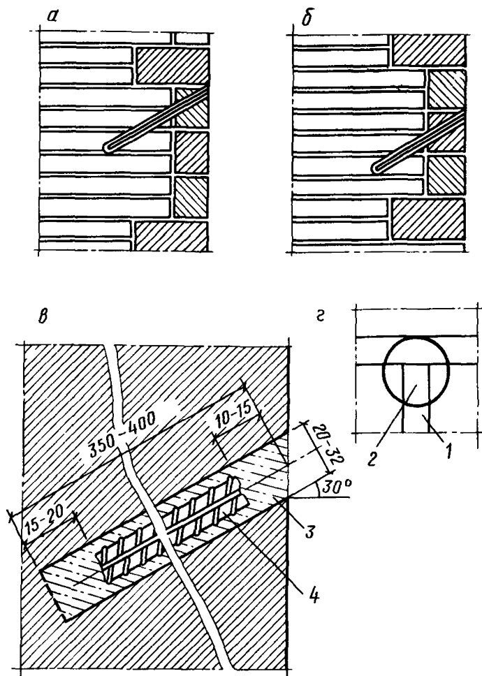
Рис. 16. Заделка стержней в кладку для крепления облицовки
