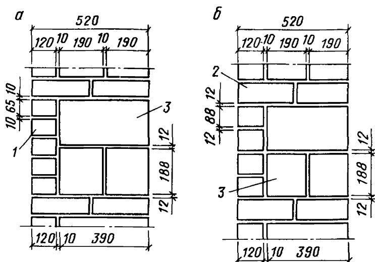
Рис. 4. Облицовка лицевым кирпичом стен из бетонных камней
