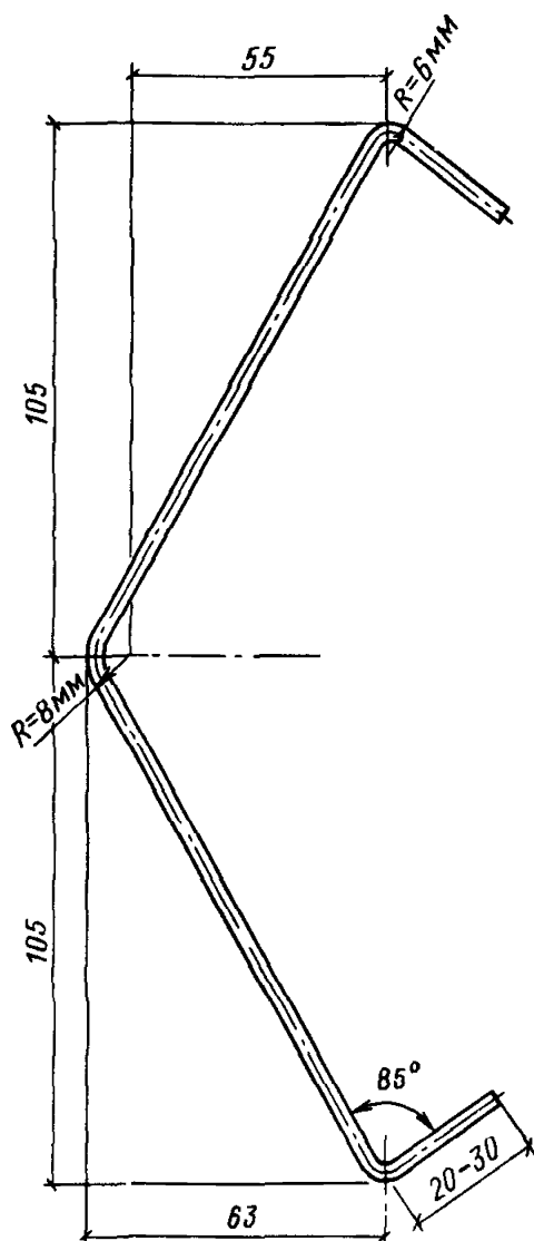
Рис. 13. Пружинная закрепа
