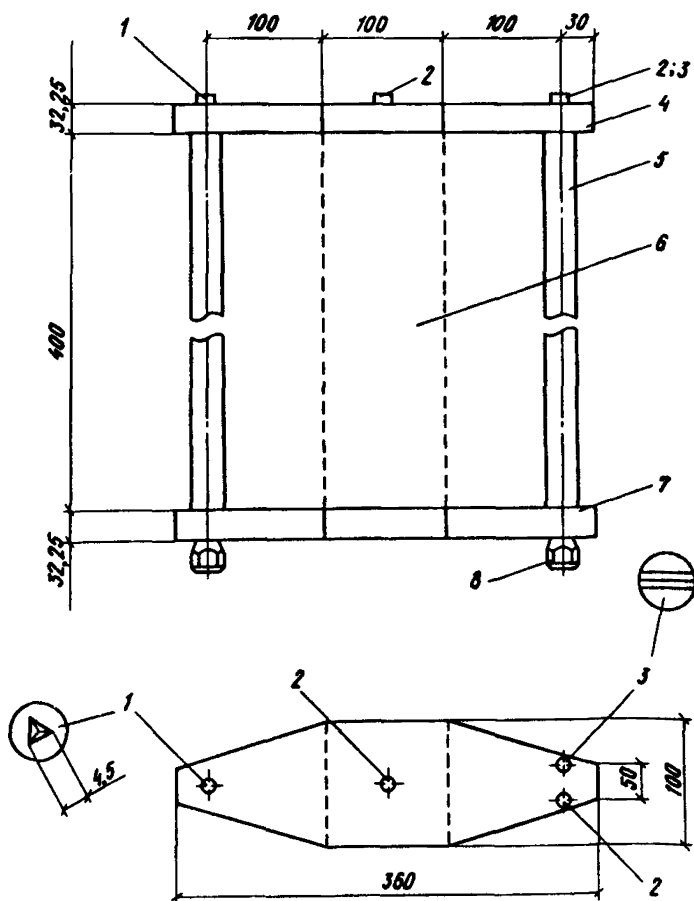
Рис. 2. Динамометрический кондуктор для образцов-призм размером 10х10х40 см
