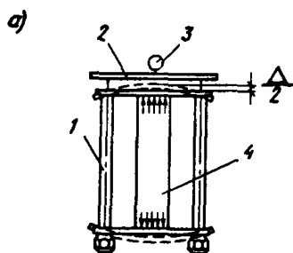
Рис. 3. Измерительное устройство "краб" с индикатором часового типа
