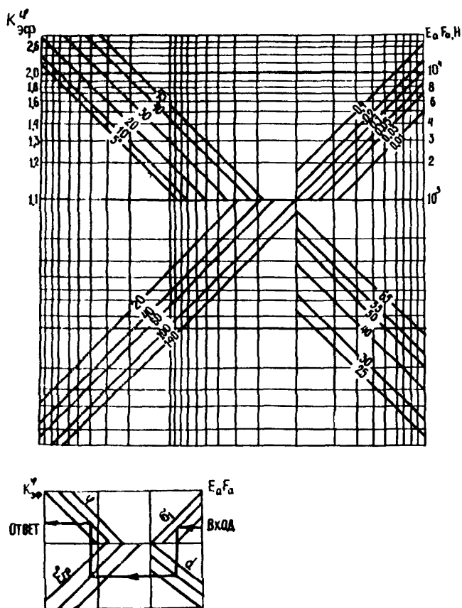
Рис.3. Номограмма для определения коэффициента эффективности армирования K_{эф.д}^{\psi} — средняя крупность зерен материала основания (покрытия) в зоне контакта с подстилающим грунтом, определяемая как среднее арифметическое между верхним и нижним пределами фракции щебня, мм; \psi — угол внутреннего трения грунта, подстилающего щебеночный слой, град.
