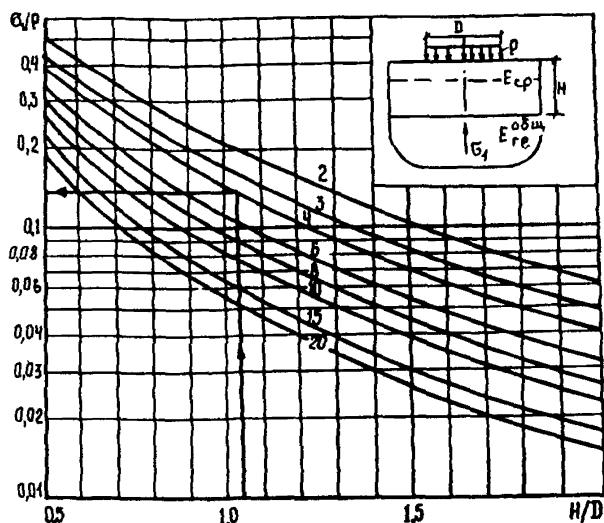
Рис.2. Номограмма для определения вертикального главного напряжения на уровне сетки (цифры на кривых — E_{ср}/E_{гр}^0 )
