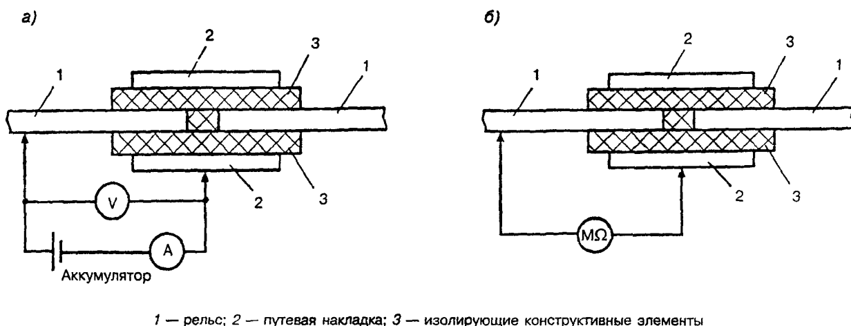
Рисунок 5 — Схема измерения сопротивления изоляции стыка ходового рельса
