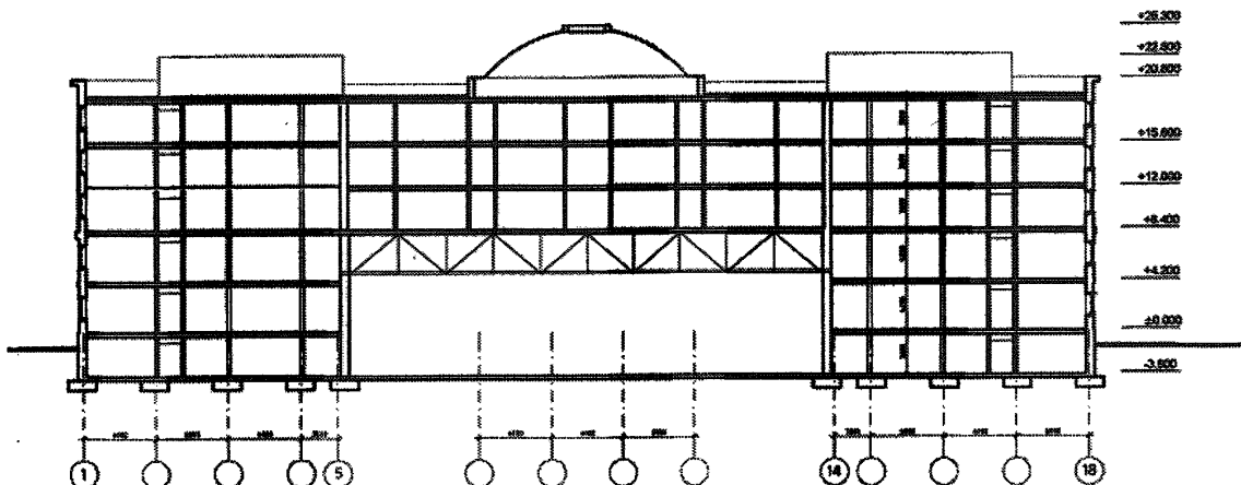
Рисунок Я.3 — Продольный разрез
