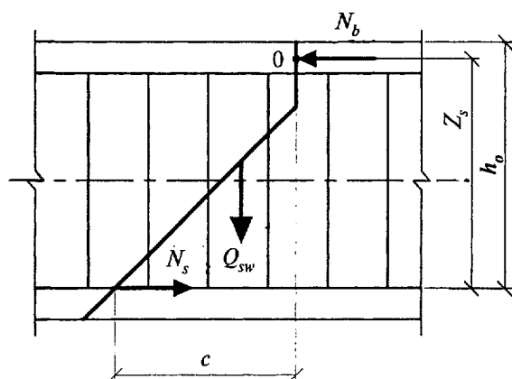
Рисунок 8 — Схема усилий при расчете изгибаемых предварительно напряженных элементов по наклонному сечению на действие моментов
