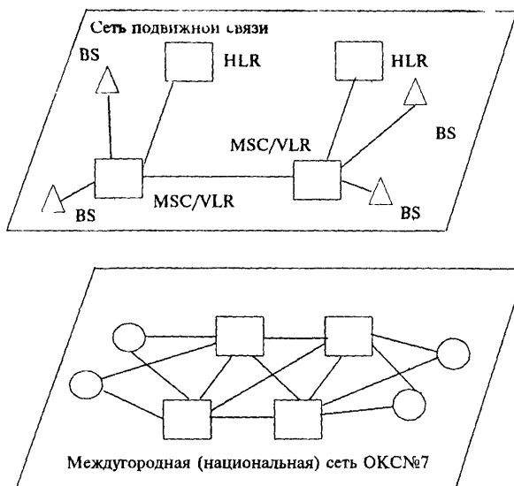
Рис 4. Построение сети ОКН№7 СПС
