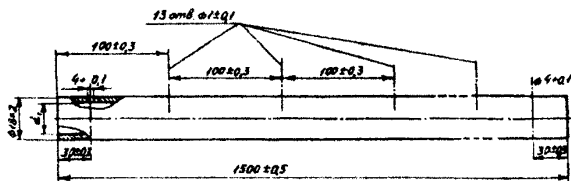
Рисунок Д.4.4 – Звено штанги
