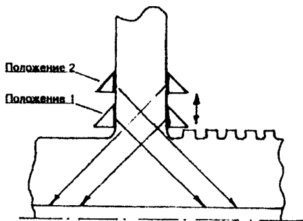
Рисунок К.8 – Схема прозвучивания ротора с поверхностей дисков
