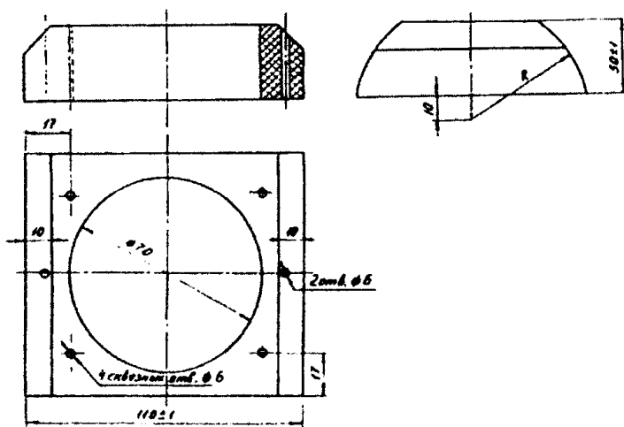
Рисунок Д.4.2 – Прижимная рамка
