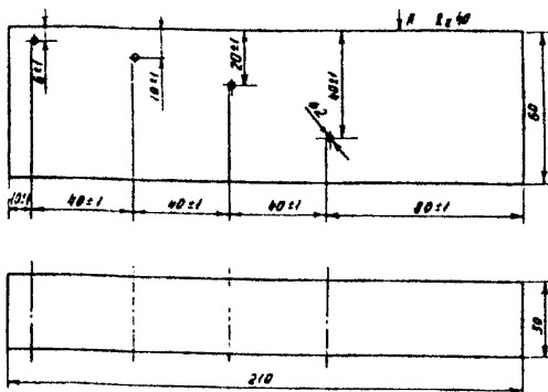
Рисунок Д.5 — Упрощенный испытательный образец
