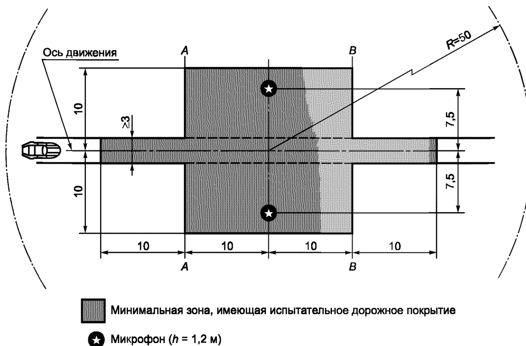
Рисунок И.1 — Минимальные требования в отношении зоны с испытательным покрытием. Затемненная часть называется испытательной зоной
