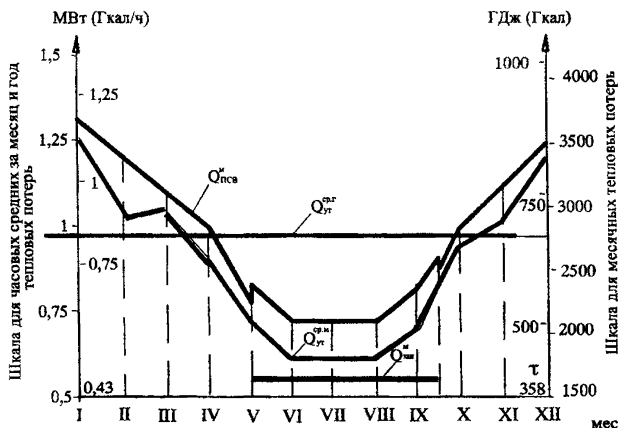
Рис. 3. Нормируемые тепловые потери с потерями сетевой воды (утечкой и на заполнение):
