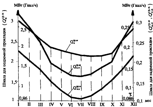
Рис. 2. Нормируемые часовые тепловые потери через теплоизоляционные конструкции при среднемесячных условиях:
