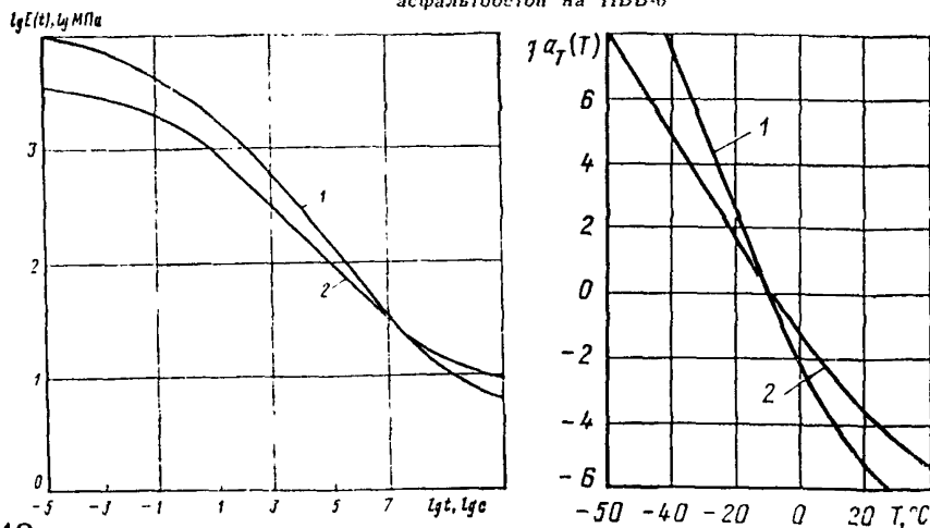
Рис. 2. Обобщенная функция релаксации E(t) при -10^\circ\text{C} и функция температурно-временного смещения a_T(T) :
