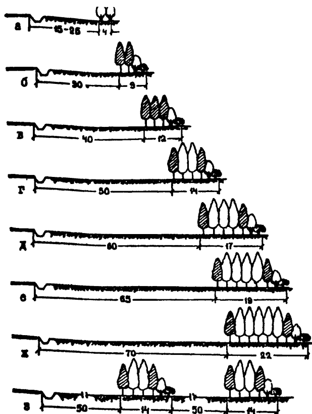
Рис. 3.1. Типовые схемы снегозащитных лесных насаждений вдоль автомобильных дорог при объеме снегопереноса ( \text{м}^3/\text{м} ).
