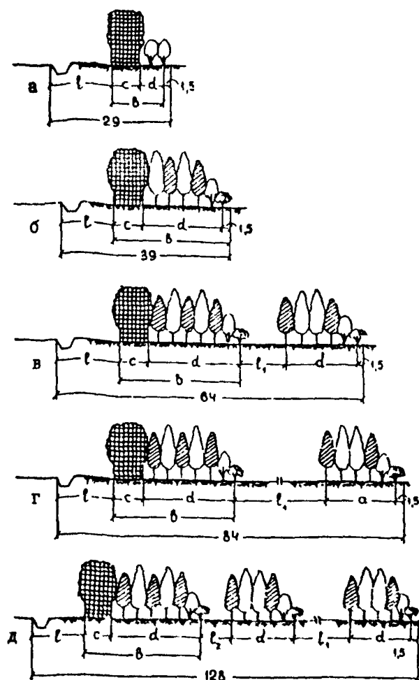
Рис. 3.3. Типовые схемы усиления существующих снегозащитных лесных насаждений вдоль автомобильных дорог при объеме снегоприноса (м 3 /м): а - до 25; б - до 50; в - до 100; г - до 150; д - до 250.
