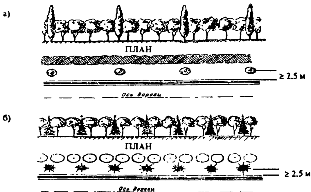
Рис. 3.6 Примеры декоративного озеленения автомобильных дорог (регулярный способ).
