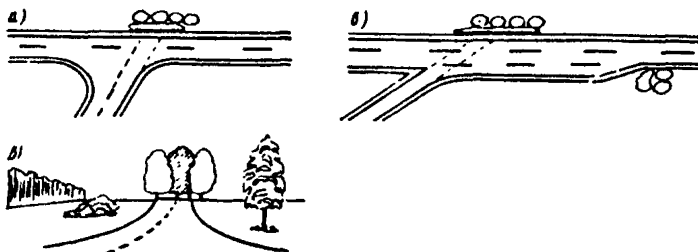
Рис. 3.11. Примеры барьерных посадок на примыканиях дорог: а - напротив съезда; б - в конце переходно-скоростной полосы; в - за выпуклой вертикальной кривой.
