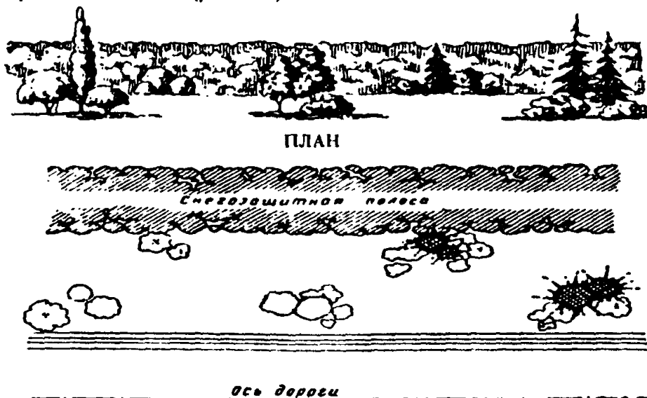
Рис. 3.8. Ландшафтно-групповой способ декоративного озеленения автомобильных дорог.
