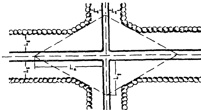
Рис. 3.2. Схема расположения лесных полос для обеспечения видимости на пересечениях автомобильных дорог.
