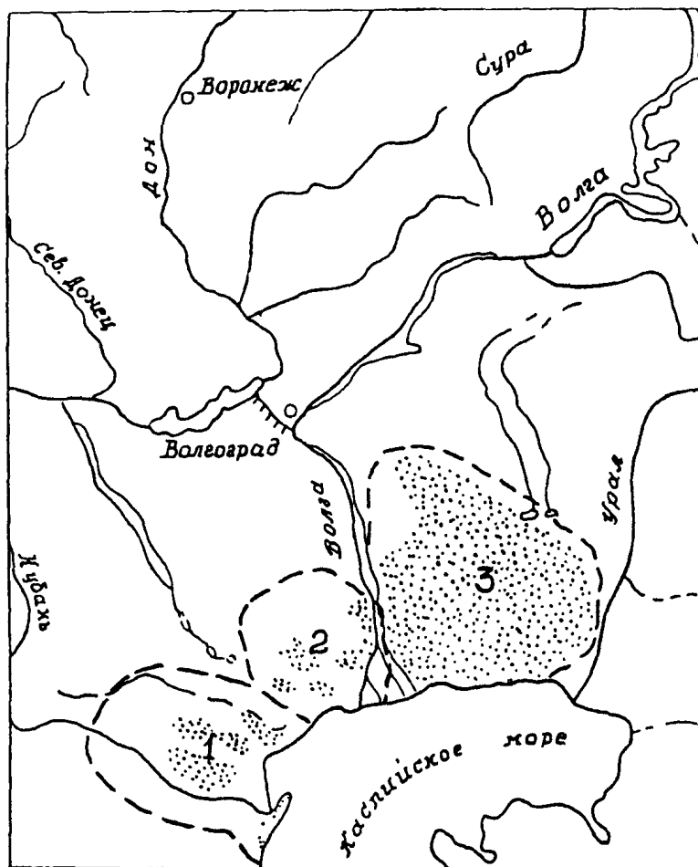
Рис. 3.4. Схема основных песчаных массивов на территории Российской Федерации.
