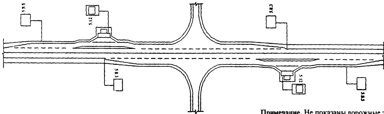
Рис. Б.4. Расстановка дорожных знаков у автобусных остановок
