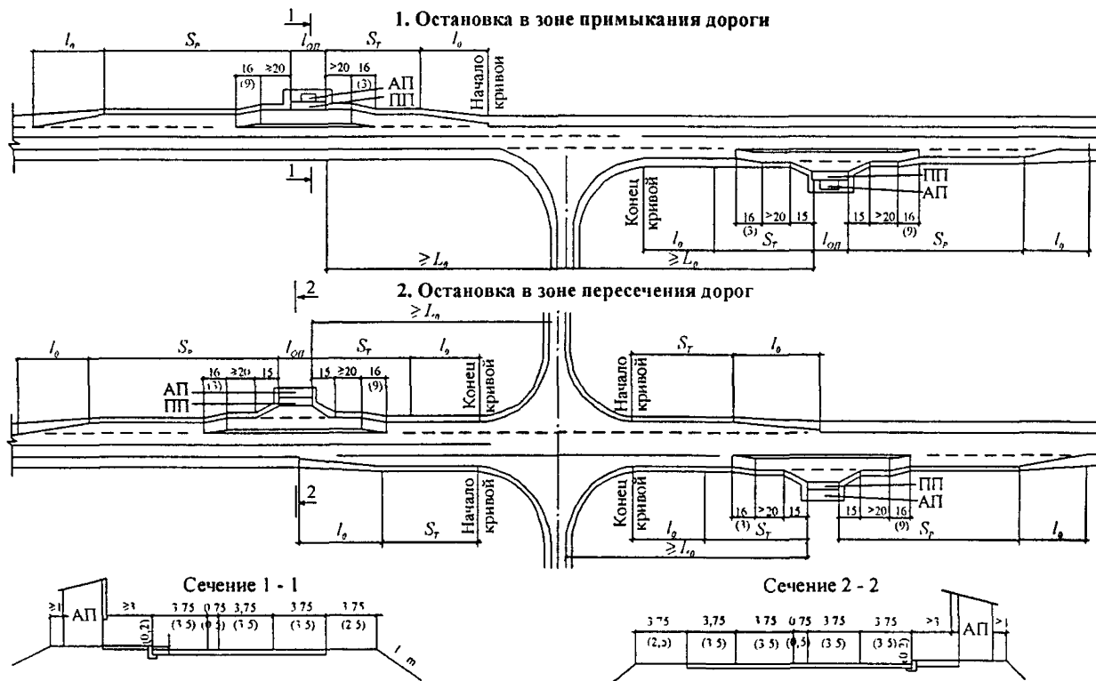
Рис. Б.3. Автобусные остановки на дорогах
