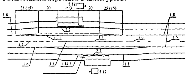
2. Разметка дорог II-III категорий с пешеходным переходом в одном уровне
