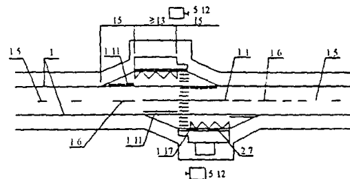
4. Разметка дорог IV категории при отсутствии переходно-скоростных полос
