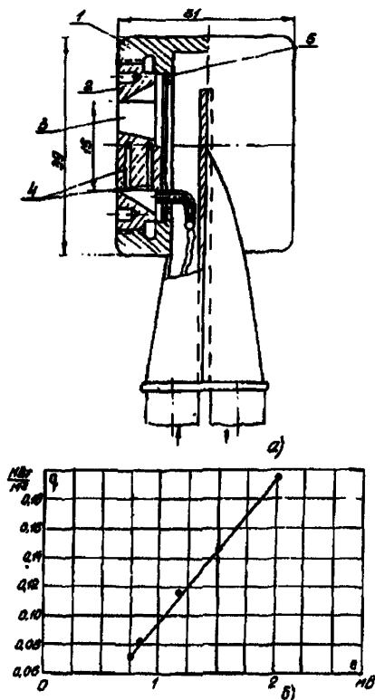
Рис.2.11. Общий вид радиационного двухстороннего термозонда (а) и его градуировочная кривая (б): 1- корпус головки; 2 - гайка нажимная; 3 - термоприемник; 4 - дифференциальный хромель-копелевый ТЭТ; 5 - прокладка
