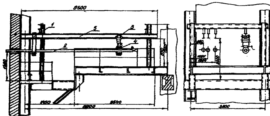
Рис.2.6. Оборудование площадки для применения и перемещения зондов: 1 - подвеска; 2 - зонд; 3 - тележка; 4 - устройство крепления и поворота зонда; 5 – монорельс (двуглав № 12-16); L=6500 мм
