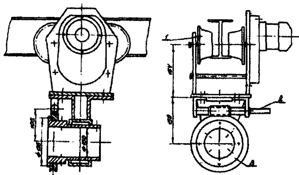
Рис.2.4. Приспособление для перемещения и вращения зонда:
