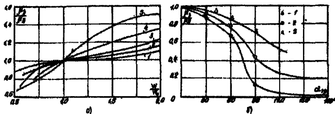
Рис.2.9. Влияние скорости отсоса (а) и угла наклона головки зонда к направлению потока (б) на концентрацию пыли: диаметр частиц, мкм: 1-4; 2-12; 3-17; 4-31; 5-37
