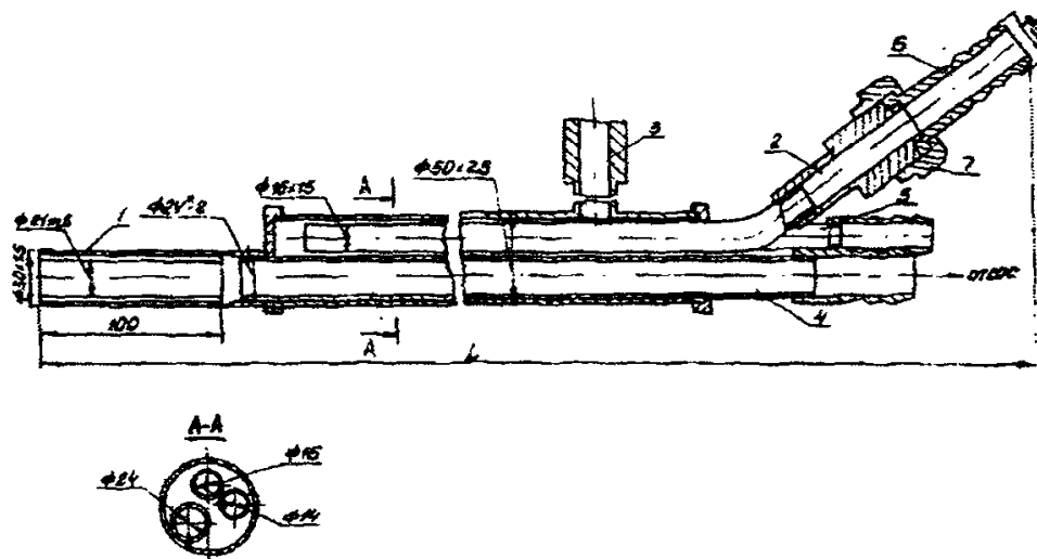
Рис.2.2. Зонд водоохлаждаемый для отсосного ТЭТ и отбора проб газов: 1 - съемный насадок; 2 - канал для подвода воды; 3 - канал для отвода воды; 4 - канал для отбора газов; 5 - канал для установки ТЭТ; 6 - штуцер; 7 - гайка накидная, L=3000+6000 мм
