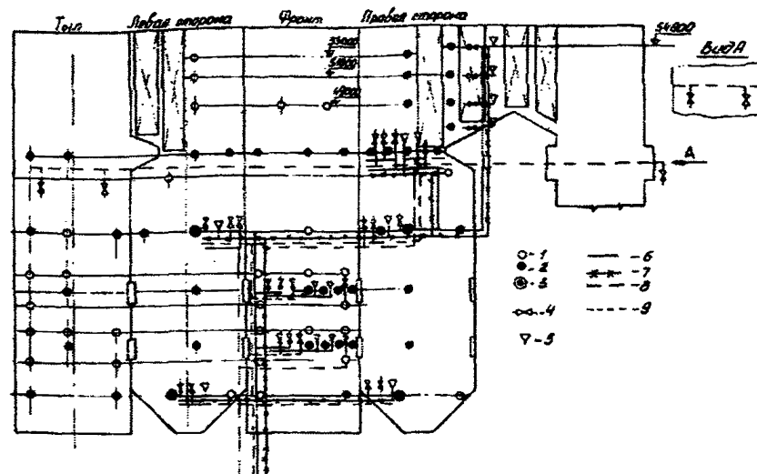
Рис.2.1. Схема расположения дополнительных лючков, трубопроводов воды, сжатого воздуха, отсоса газов и сброса воды котла ТПЕ-214:
