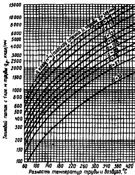
Рис. 13. Номограмма для определения тепловых потерь неизолированными поверхностями
