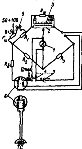
Рис. 11. Принципиаль-схема термощупа ОРГРЭС Т-4
