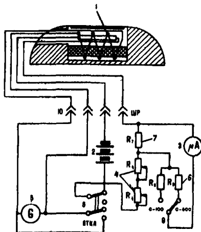
Рис. 4. Схема вторичного прибора
