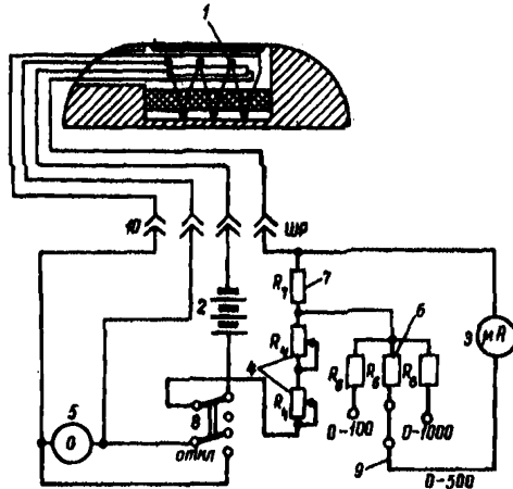
Рис.8. Схема прибора с дополнительным диапазоном измерения
