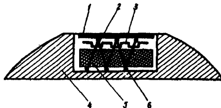
Рис.2. Схема датчика тепломера
