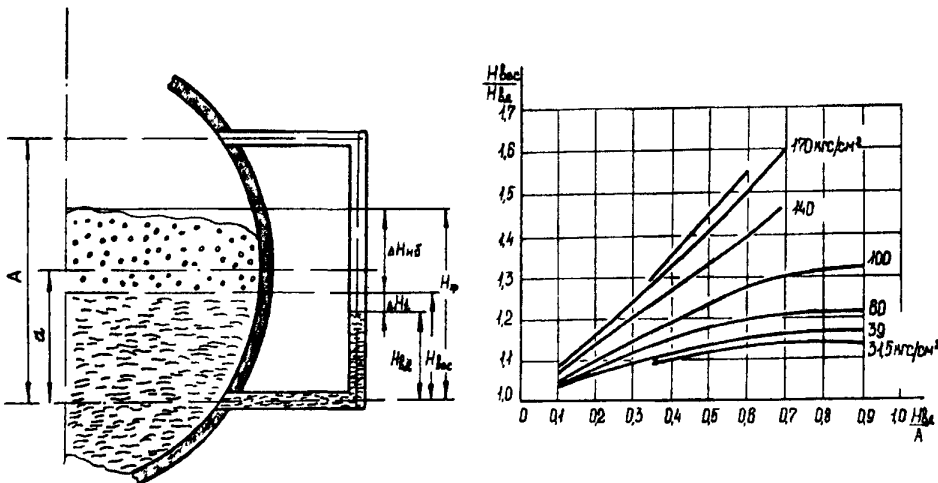
Рис. 12. Поправка на охлаждение воды в водоуказательной колонке
