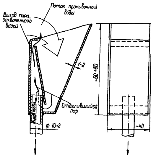
Рис. 11. Зонд для отбора проб промывочной воды
