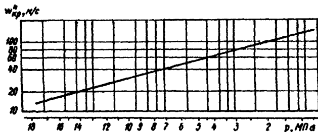
Рис. 3. Зависимость критической скорости пара срыва пленки влаги от давления
