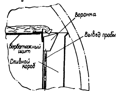
Схема установки воронки
