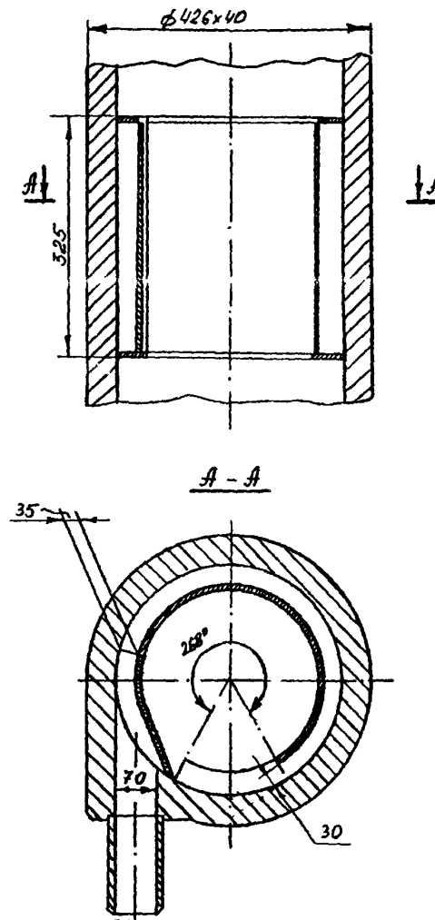
Рис. 21. Улитка выносных циклонов котла ТП-230-2
