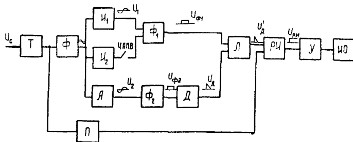
Рис.ПІ.І. Структурная схема реле частоты
