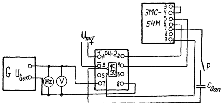
Рис.5.4. Схема проверки времени срабатывания реле PC-2
