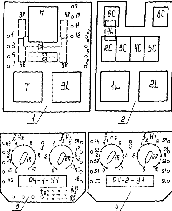
Рис. 4.1. Схема расположения элементов реле частоты: 1 - основание корпуса; 2 - откидная плата; 3 - лицевая панель PC-1; 4 - лицевая панель PC-2
