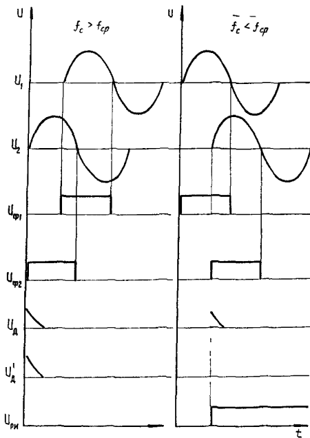
Рис.П.1.2. Время-импульсные диаграммы реле частоты
