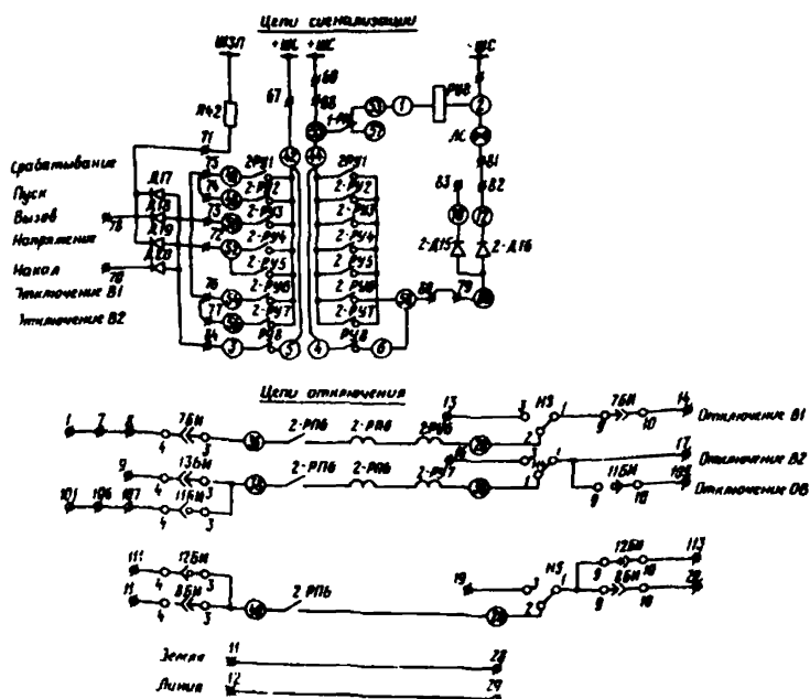
Рис. 4. Цепи постоянного тока защиты ДЗ-201:
