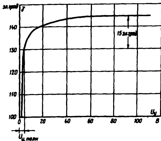
Рис. 8. Кривая зависимости длительности импульсов тока на выходе приемника от значения напряжения U_y
