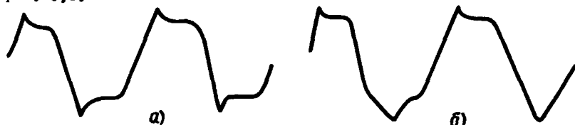
Рис. 6. Форма кривой напряжения на стабилизаторах органа управления: а - при правильной полярности обоих стабилизаторов; б - при неправильной их полярности
