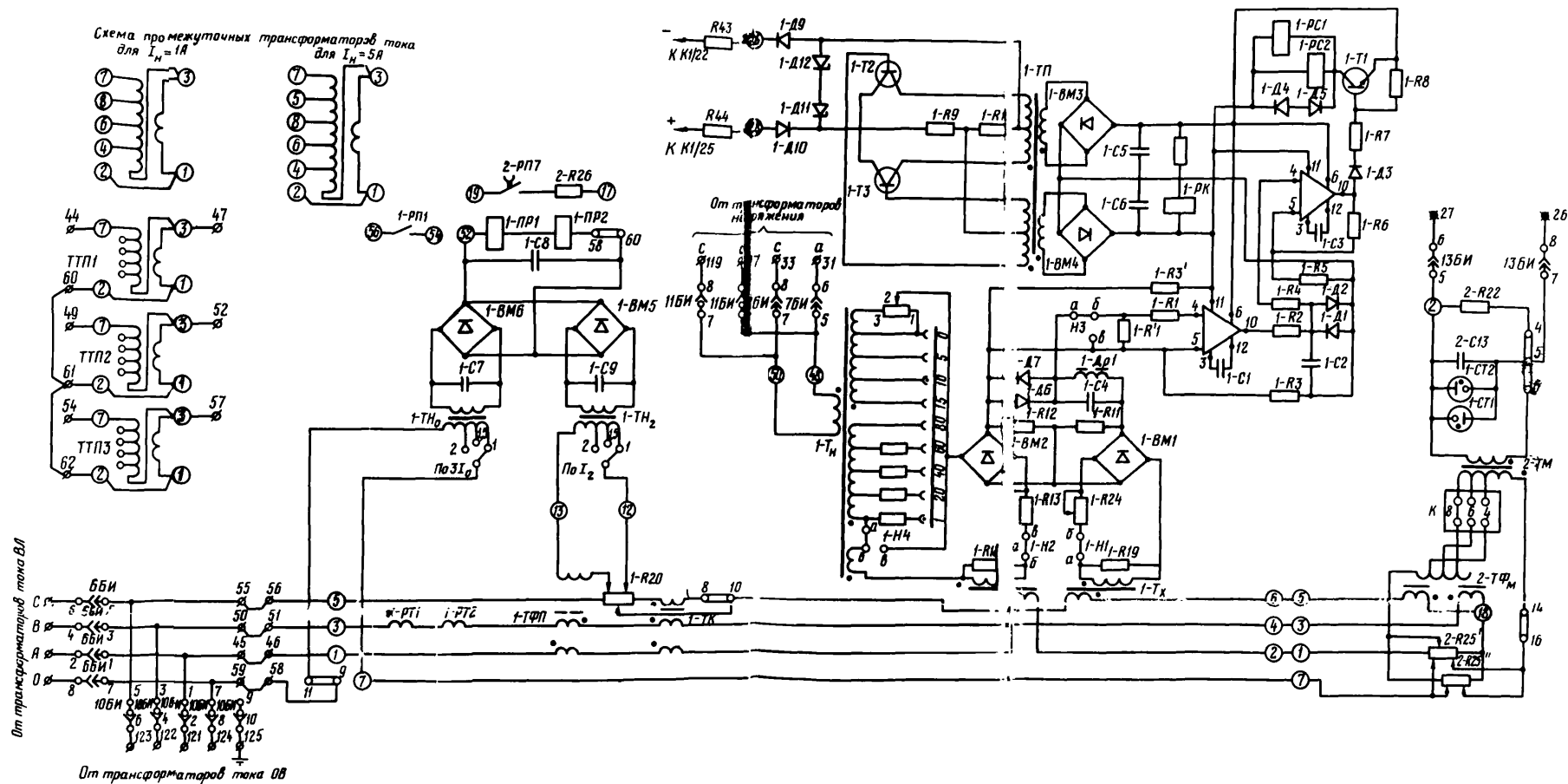
Рис. 3. Цепи переменного тока и напряжения защиты ДЭС-201
