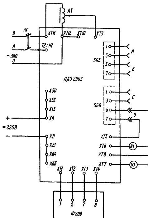
Рис.9. Схема проверки панели ПДЗ 2002 от встроенного проверочного устройства
