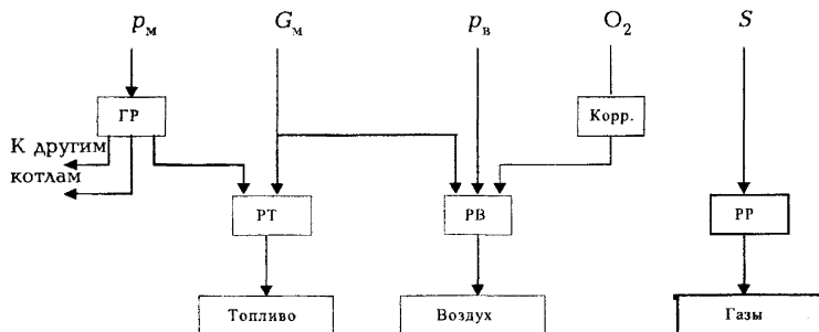
Рис. 1. Типовая схема регулирования нагрузки барабанного котла:
