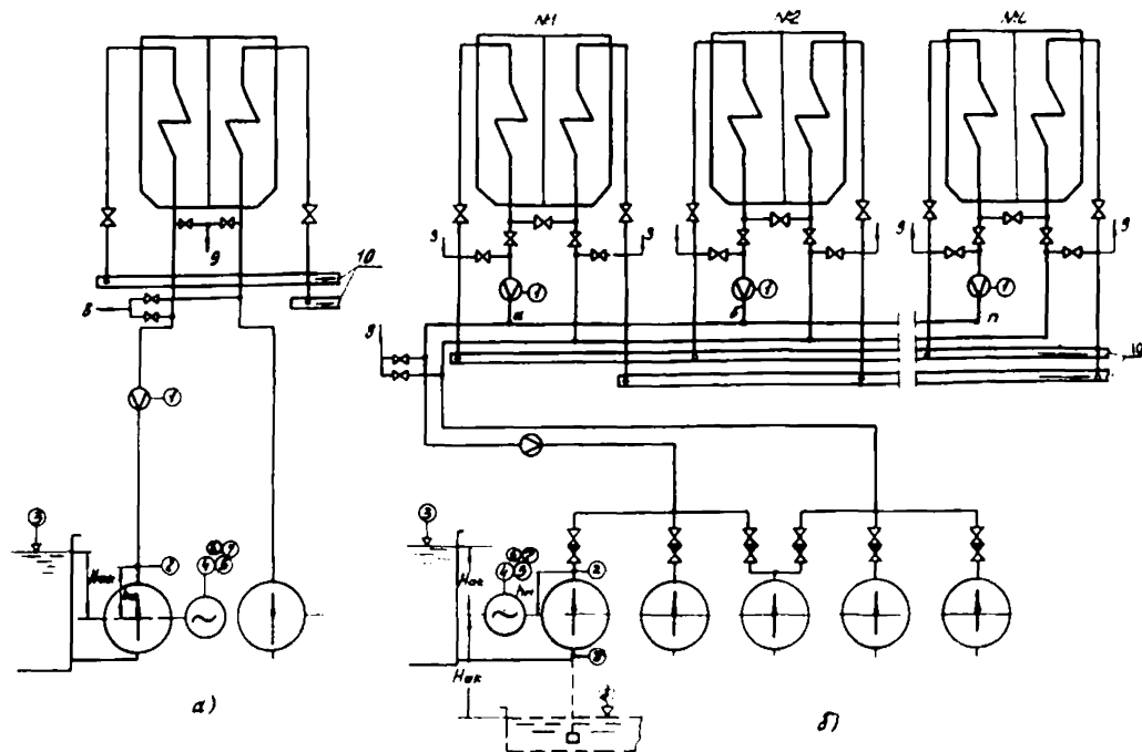
Рис. 3. Схемы технического водоснабжения конденсаторов турбин:
