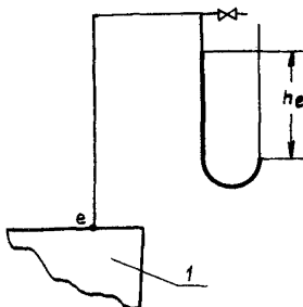
Рис. 7. Измерение разрежения в точке e с помощью ртутного вакуумметра:
