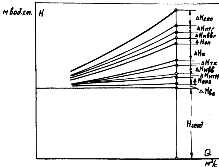
Рис. 10. Гидравлическая характеристика тракта циркуляционной воды при схеме водоснабжения с магистральными водоводами и баженными градириями (см. рис. 9)
