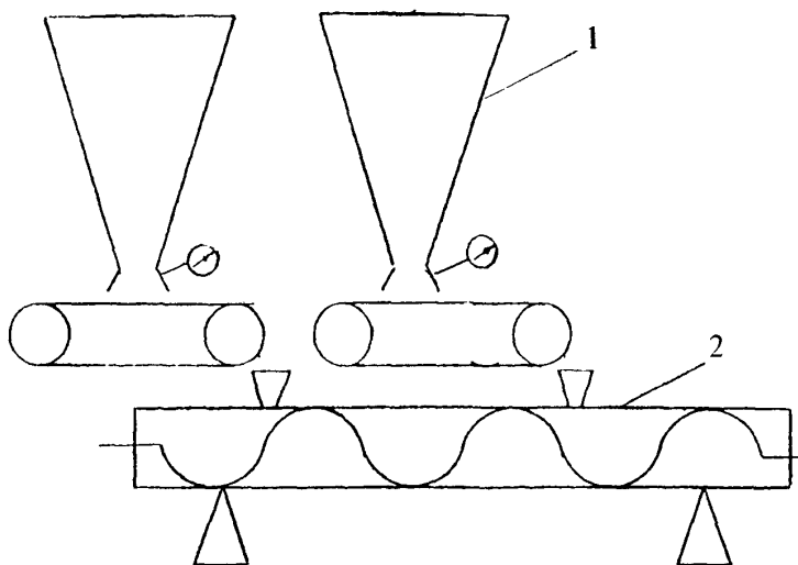
Рис. П.2.1. Схема установки для смешивания минеральных материалов: 1 - весовой дозатор; 2 - шнековый транспортер
