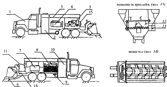
Рис. 4.1. Схема смесителя-распределителя «MACROPAVER»:
