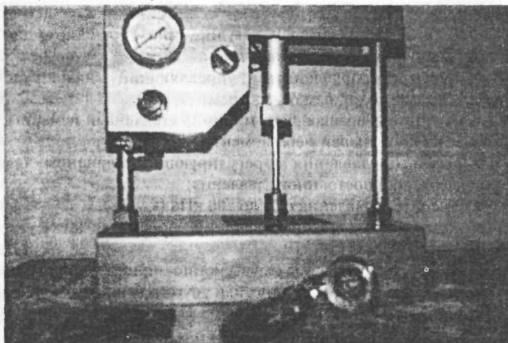
Рис. П.4.1. Модифицированный определитель силы сцепления
