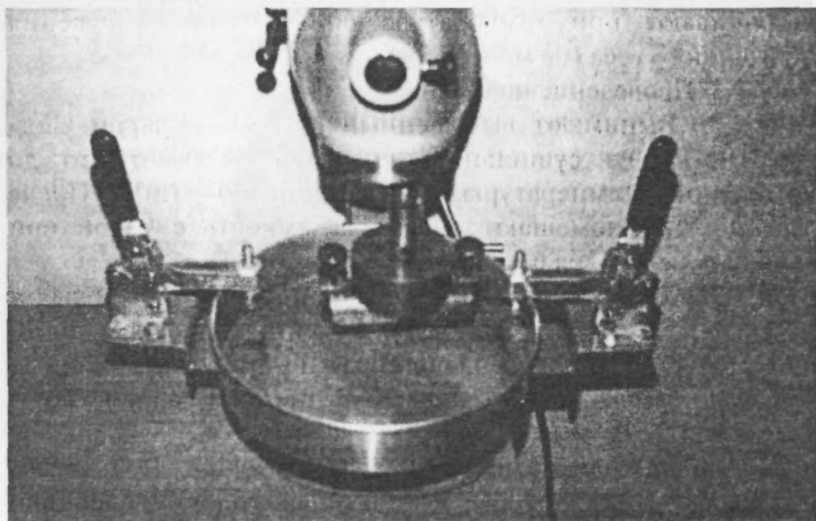
Рис. П.5.1. Прибор для определения мокрого истирания
