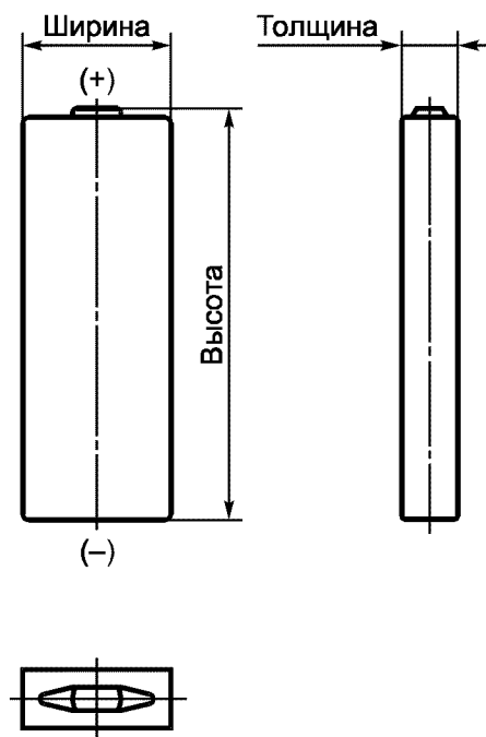
Рисунок 2 — Малогабаритный призматический аккумулятор
