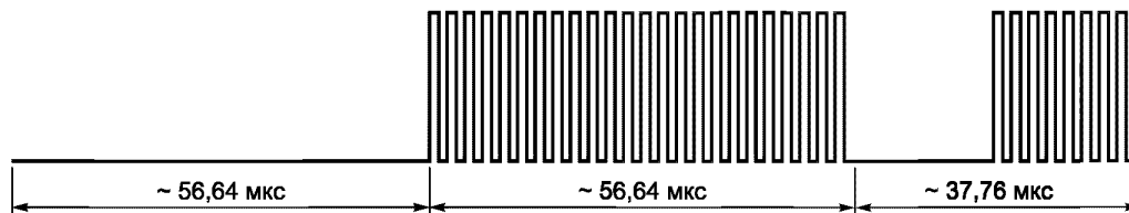
Рисунок 14 — Начало кадра при использовании одной поднесущей
