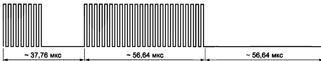
Рисунок 16 — Конец кадра при использовании одной поднесущей
