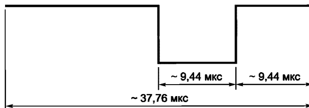
Рисунок 9 — Конец кадра при любом способе кодирования
