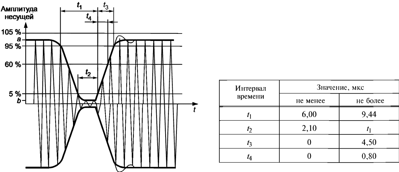
Рисунок 1 — Модуляция несущей для случая 100 % ASK
