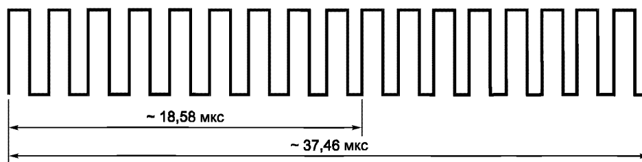
Рисунок 13 — Логическая единица
