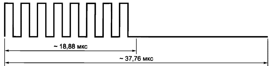
Рисунок 10 — Логический ноль
