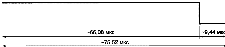
Рисунок 5 — Способ кодирования «1 из 4»
