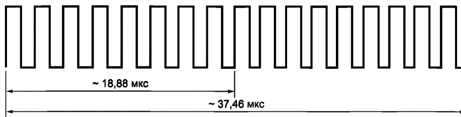
Рисунок 12 — Логический ноль
