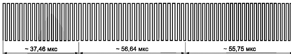
Рисунок 17 — Конец кадра при использовании двух поднесущих
