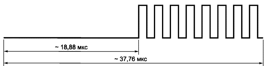
Рисунок 11 — Логическая единица
