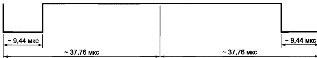
Рисунок 7 — Начало кадра при способе кодирования «1 из 256»
