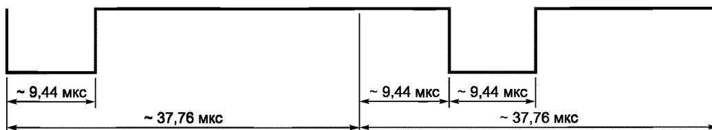
Рисунок 8 — Начало кадра при способе кодирования «1 из 4»
