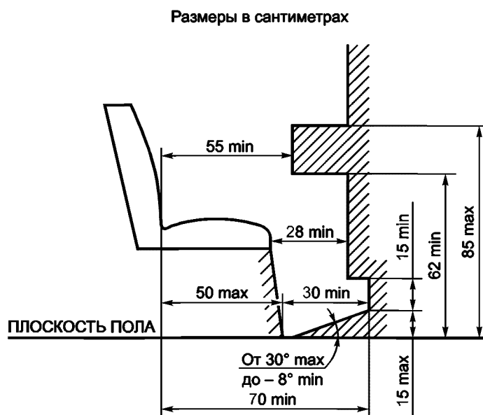
Рисунок Г.8 — Пространство для сидящих пассажиров (см. 5.7.8.5)
