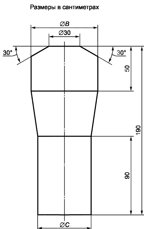
Рисунок Г.3 — Проходы (см. 5.7.5)
