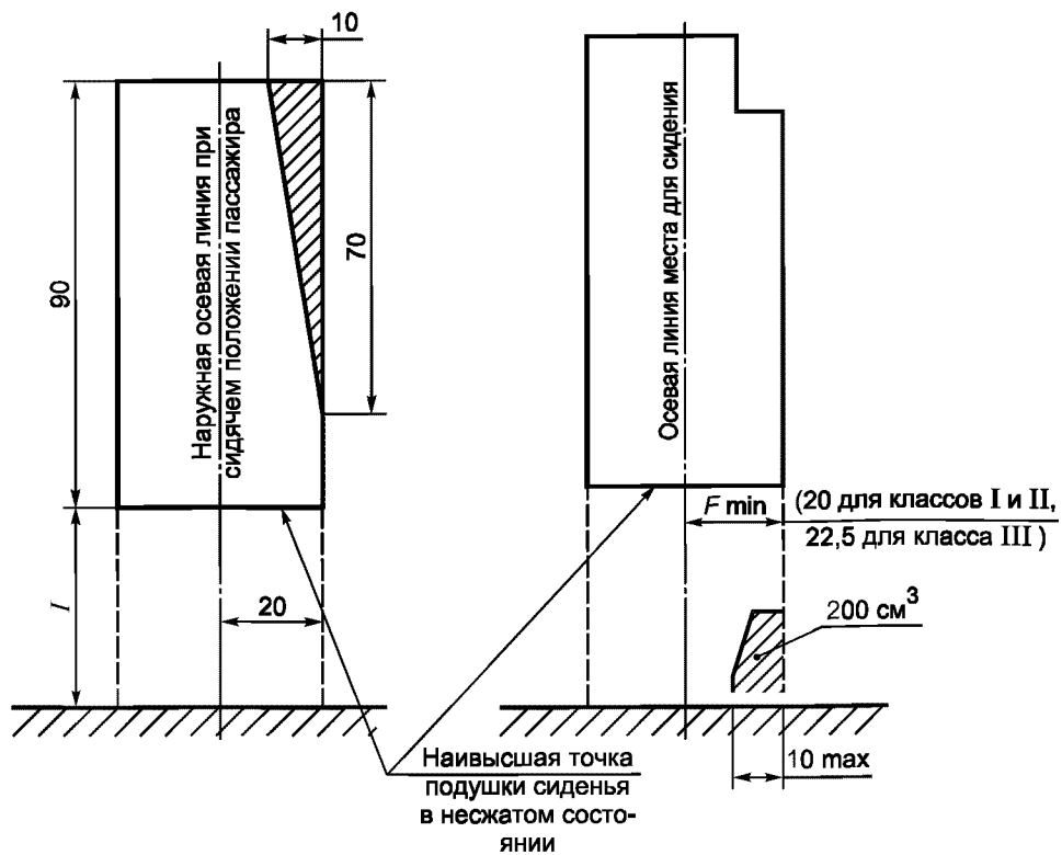
Рисунок Г.10 — Допустимый выступ элемента конструкции (см. 5.7.8.6.2.2)
