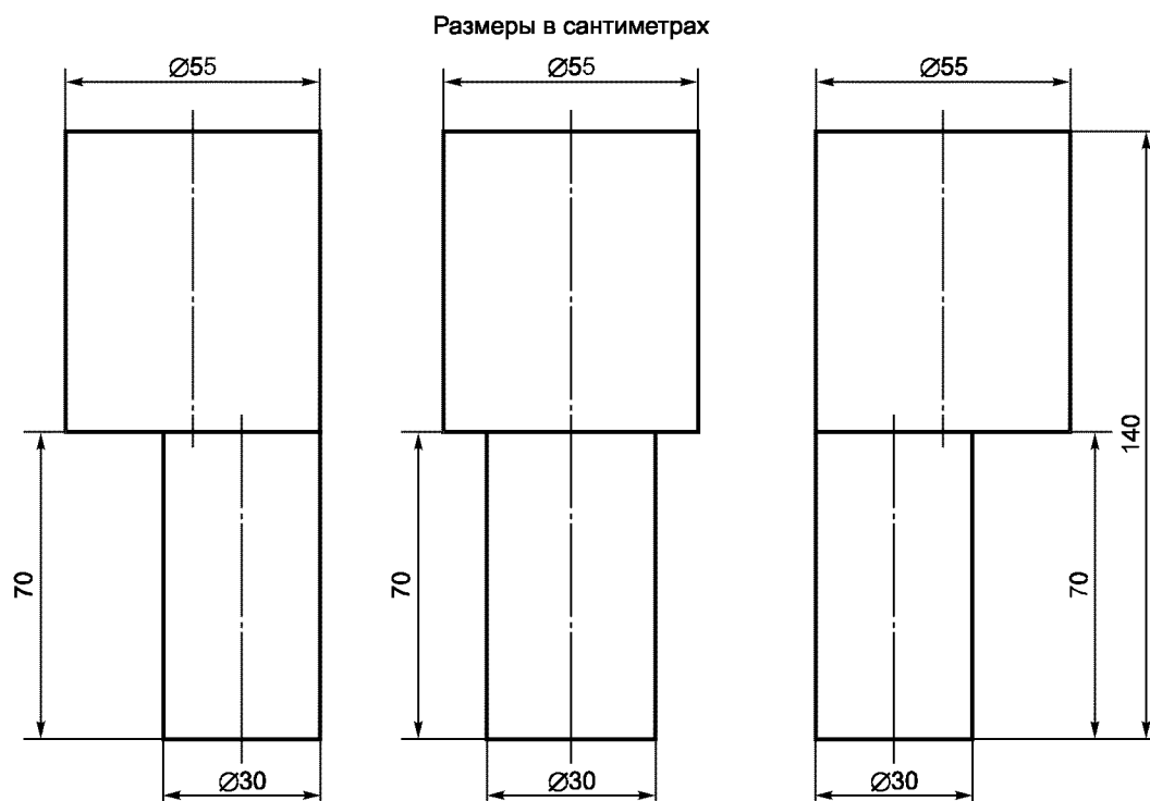
Рисунок Г.2 — Доступ к запасным дверям (см. 5.7.2)
