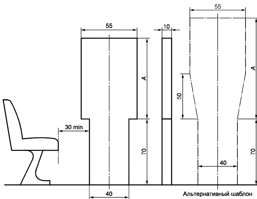
Рисунок Г.1 — Доступ к служебным дверям (см. 5.7.1)
