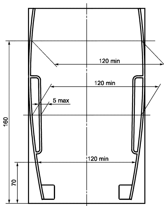
Рисунок Г.12 — Проем служебной двери. Сдвоенная дверь (см. 5.6.3.1)
