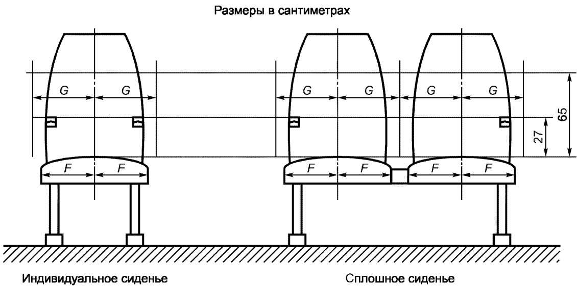
Рисунок Г.5 — Ширина пассажирских сидений (см. 5.7.8.1)
