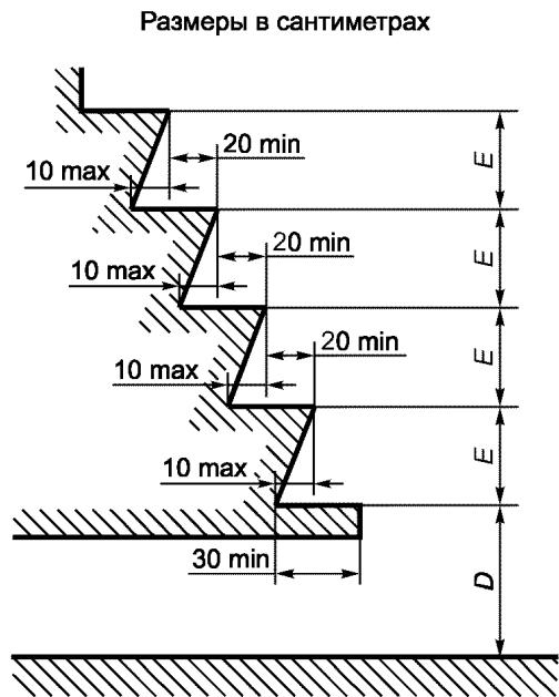
Рисунок Г.4 — Ступеньки для пассажиров (см. 5.7.7)
