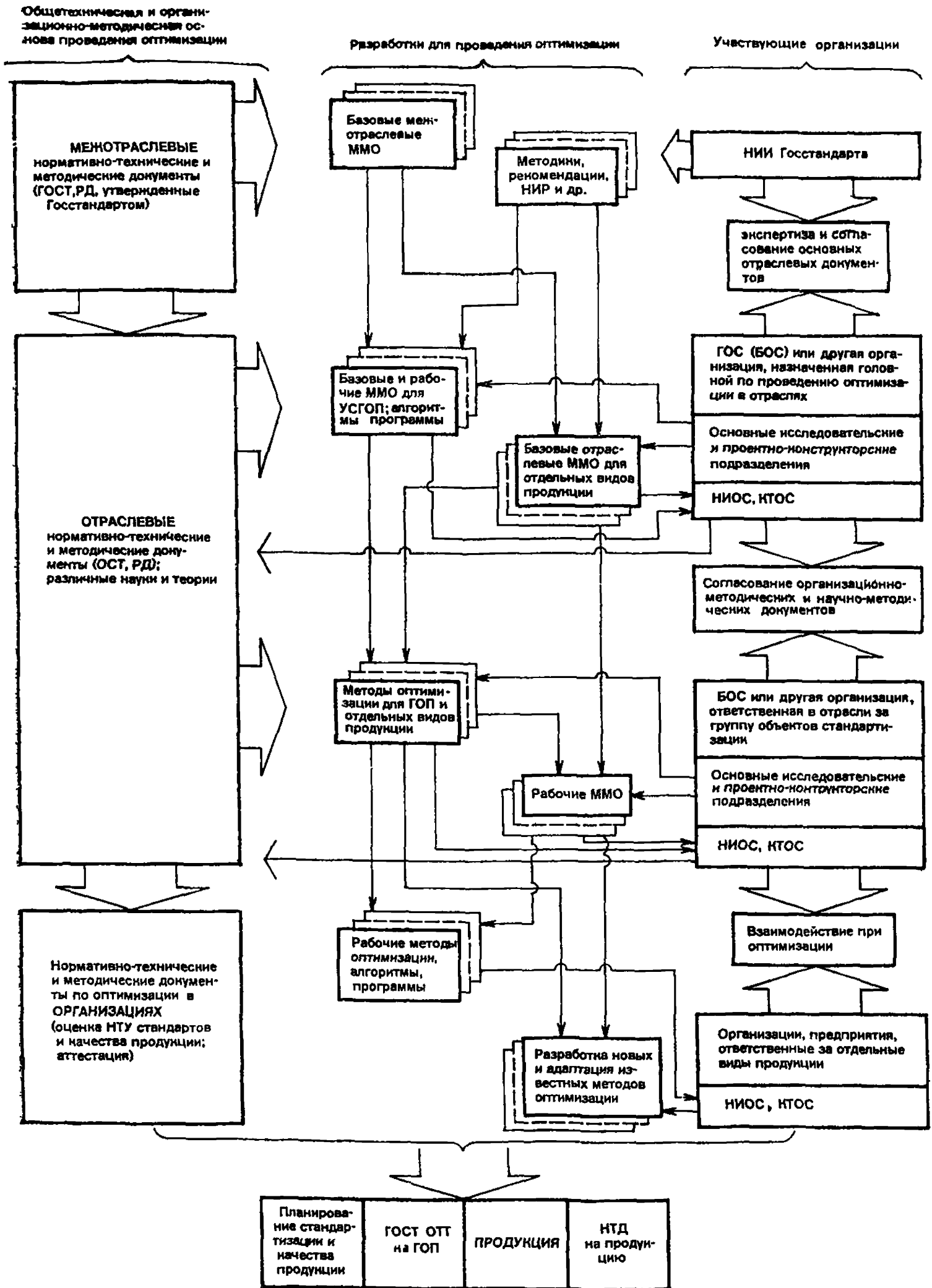
Принципиальная структурно-функциональная схема оптимизации параметров объектов стандартизации: ММО—математическая модель оптимизации; ГОП—группа однородной продукции; УСГОП—укрупненная совокупность ГОП
