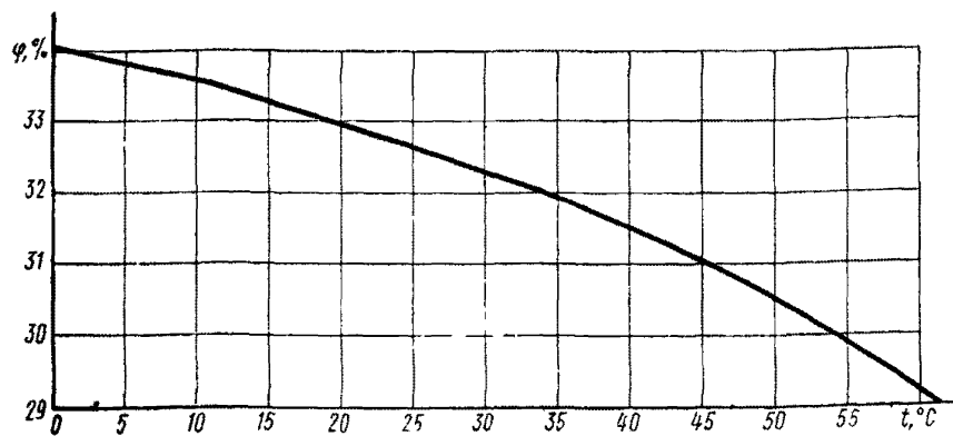
Черт. 6. График зависимости относительной влажности над раствором соли \text{MgCl}_2 от температуры
