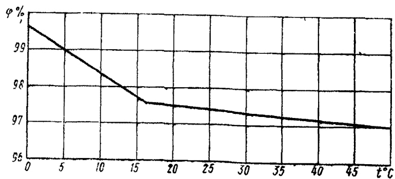
Черт 5. График зависимости относительной влажности над раствором соли \text{K}_2\text{SO}_4 от температуры
