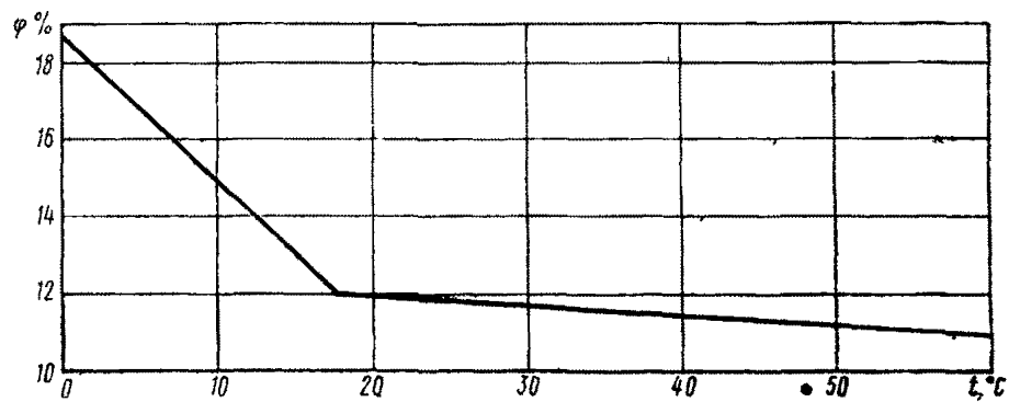
Черт 4 График зависимости относительной влажности над раствором соли LiCl от температуры
