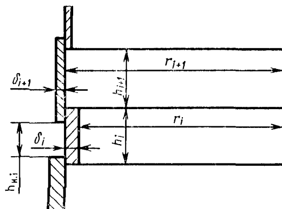
Схема поясов резервуара
