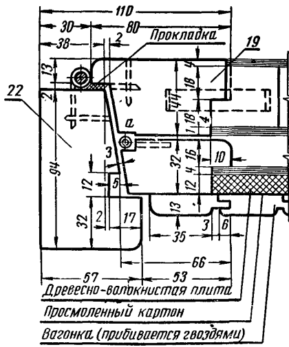
б) Сечение бокового бруска и обвязок
