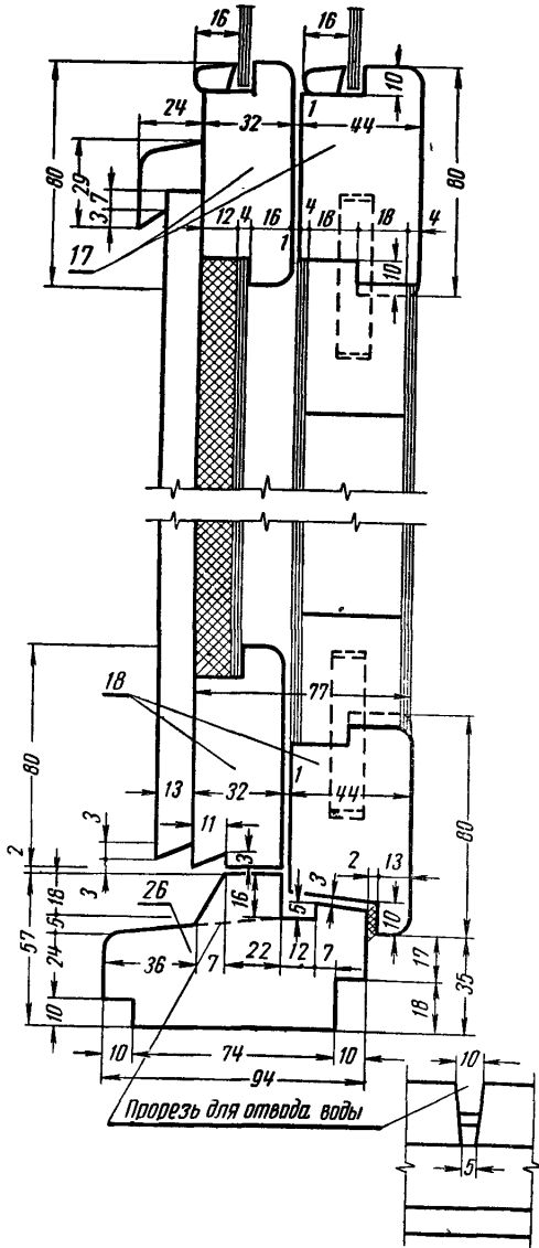
а) Вертикальное сечение нижней (глухой) части двери
