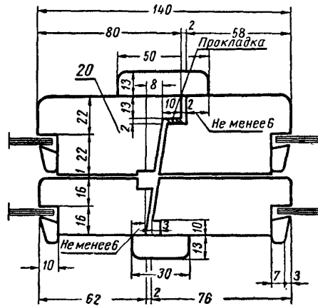
б) Притвор в глухой части дверей
