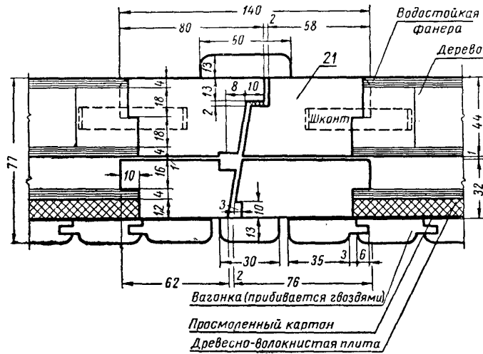
б) Притвор в глухой части дверей
