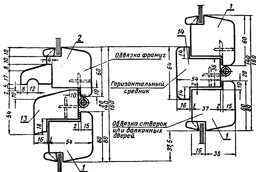
Деталь Б
