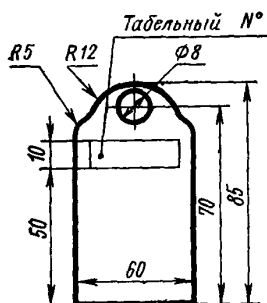
Форма 10а Чертежная марка
