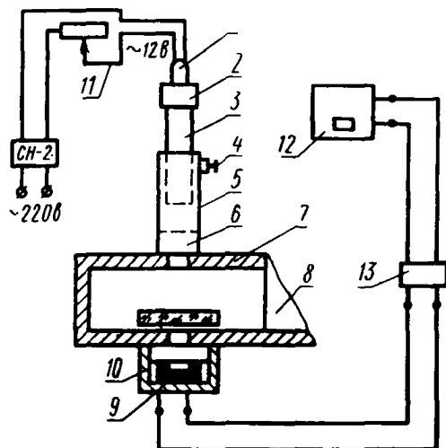
1—установочный ниппель для электропатрона; 2—лампа (12 в, 40 вт); 3—верхняя подвижная телескопическая труба; 4—верньер для перемещения верхней трубы; 5—нижняя подвижная телескопическая труба; 6—пять диафрагм с отверстиями диаметром 20—40 мм; 7—оптическая камера; 8—шторка из черного сукна; 9—вентильный селеновый элемент чувствительностью 400—550 мкА/лм; 10—камера для установки селенового фотоэлемента; 11—реостат; 12—гальванометр чувствительностью 10^{-8} — 10^{-10} а; 13—каскадный магазин сопротивлений.
