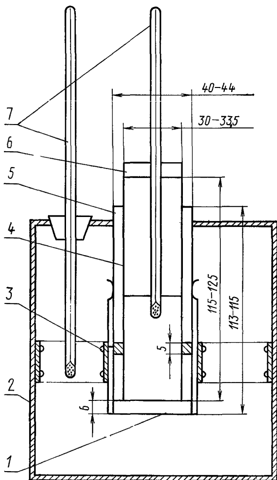
1 — диск; 2 — баня; 3 — прокладка; 4 — пробирка; 5 — муфта; 6 — корковая пробка; 7 — термометр
