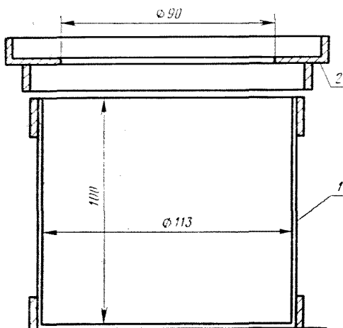
1 — стальной цилиндрический сосуд; 2 — насадка
