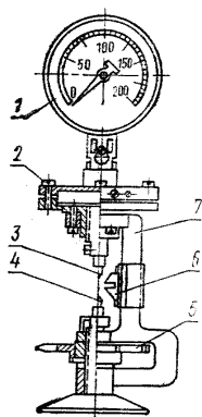
1 — манометр; 2 — гидравлическая манометр; 3 — верхний зуб; 4 — нижний зуб; 5 — щелевой упор; 6 — диск винтового механизма; 7 — корпус прибора
