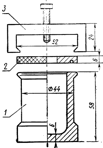
1 — корпус; 2 — крышка; 3 — захват Черт. 1
