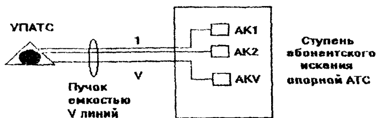
Рис. 1. включение в абонентские комплексы опорной АТС
