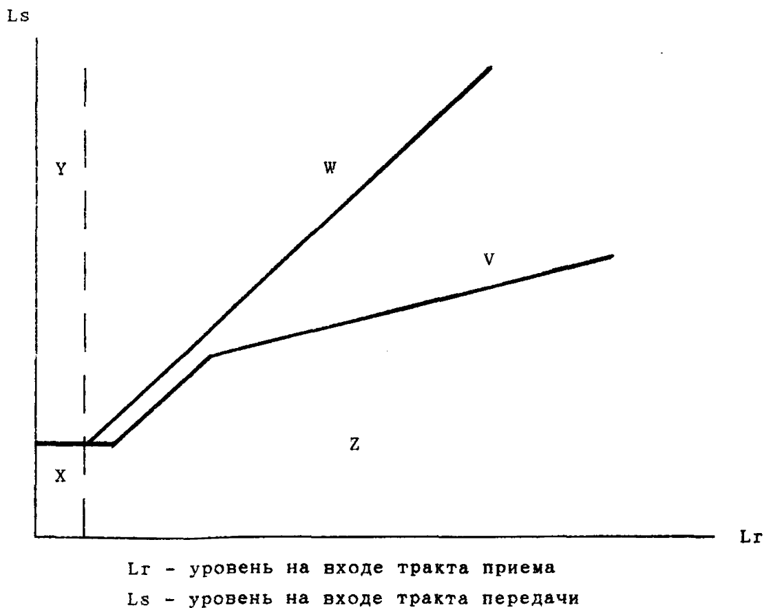
Рисунок 1 - Идеализированная диаграмма рабочих состояний ЭЗ
