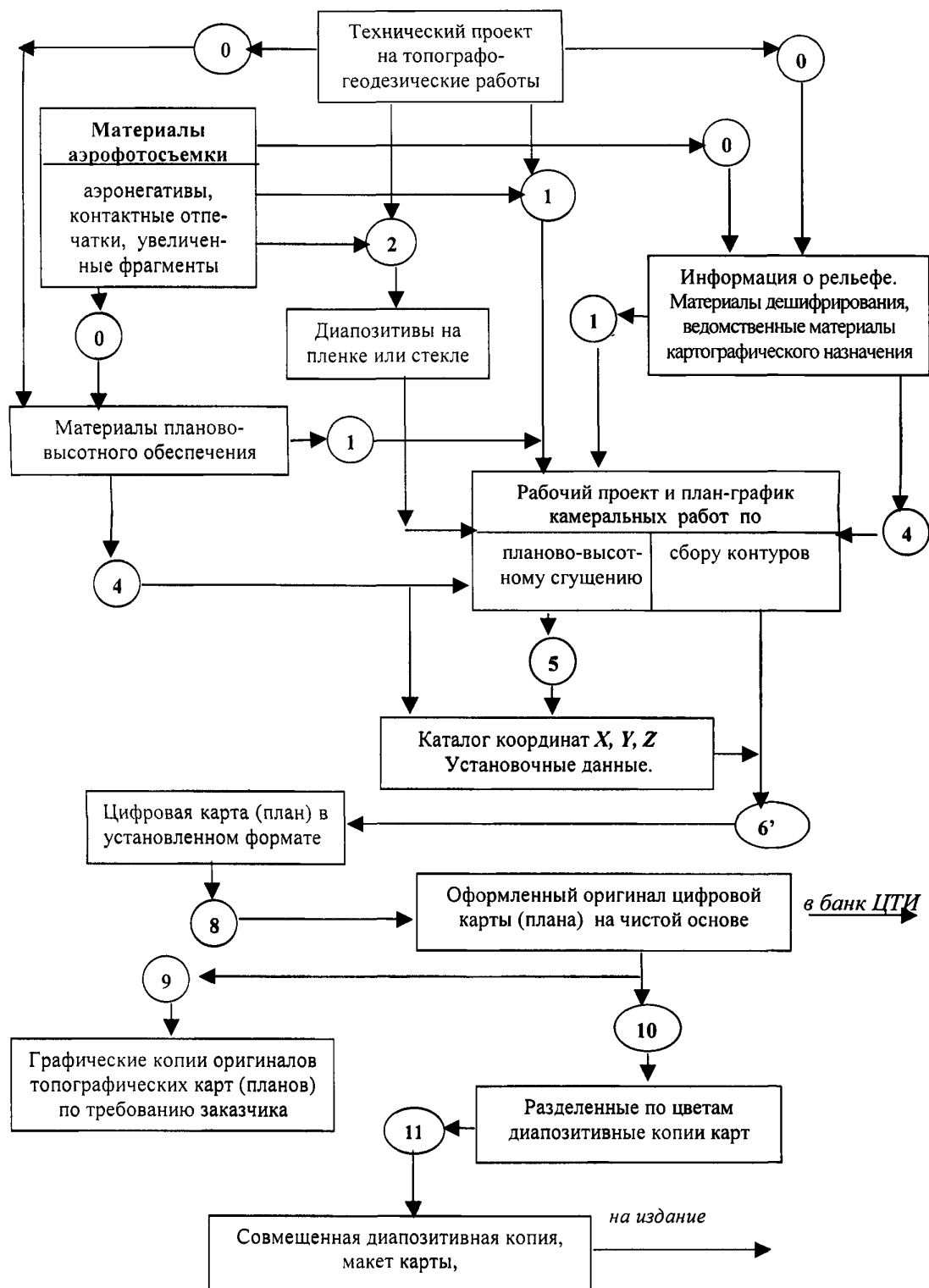
Рис. 5. Технологическая схема камеральных работ при комбинированной топографической съемке в масштабах 1:500 - 1:25000 с использованием аналитических фотограмметрических приборов
