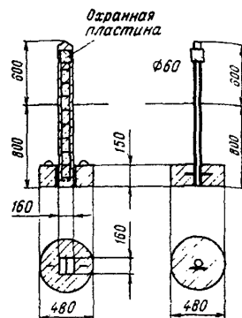
Рис. 16 Опознавательные столбы для области сезонного промерзания грунтов
