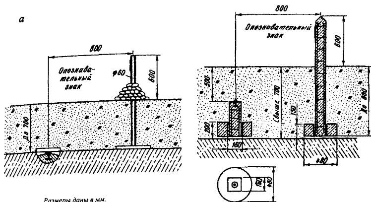
Рис. 11. Грунтовые репера для скальных грунтов: а – тип 9 оп. Знак; б – тип 176 оп. знак
