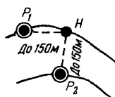
Рис. 20. Схема нивелирования через препятствие
