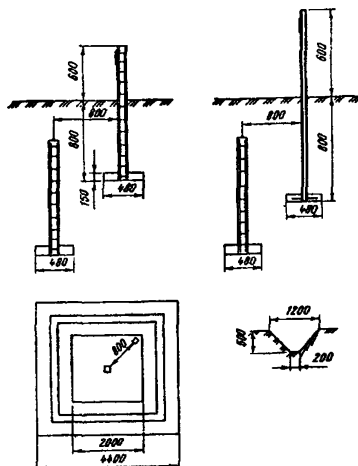
Рис. 18 Внешнее оформление грунтового репера
