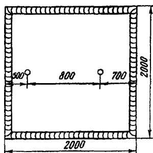
Рис. 19 внешнее оформление реперов в области многолетней мерзлоты
