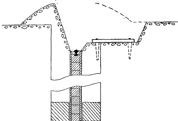
Схема установки переносной плиты
