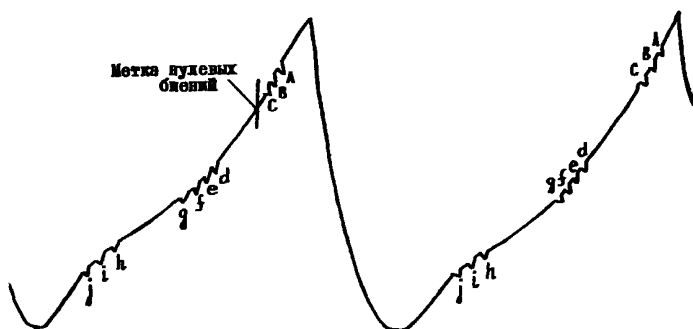
Рис. 1. Вид пиков мощности йодного лазера
