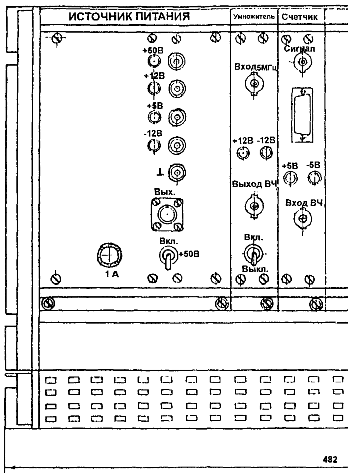
Рис.3 Лицевая панель электронно-счетного блока
