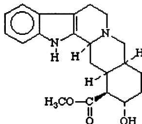
Рис. 24. Иохимбин.
