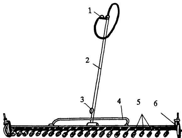
Рис. 2. Горелка воздушно-пропановая нагревательная линейная многофакельная (ГВПЛ): 1 - штуцер для присоединения запальника; 2 - ствол; 3 - запальник; 4 - распределительный коллектор; 5 - форсунки; 6 - опорные колеса
