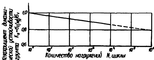
Рис.4. Зависимость коэффициента динамической устойчивости грунта от количества циклов нагружения. Песок мелкий S_z=1, \sigma_3=0,02 МПа
