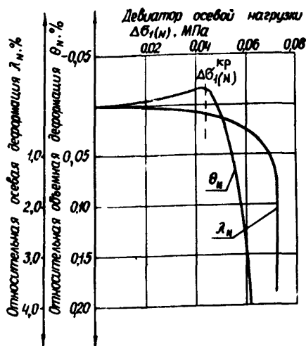
Рис.3. Закономерность деформирования грунта при повторном нагружении. Песок мелкий, \sigma_z = 1 , \sigma_3 = 0,02 МПа, f = 2 Гц, N = 10^4 циклов
