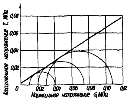
Рис.2. Диаграмма Мора. Песок мелкий, S_z = 1
